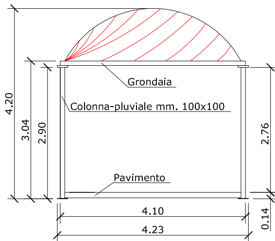
- PROSPETTO LATO 4 m
