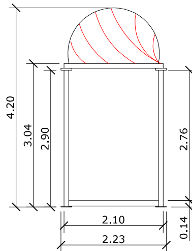
- PROSPETTO LATO 2 m
